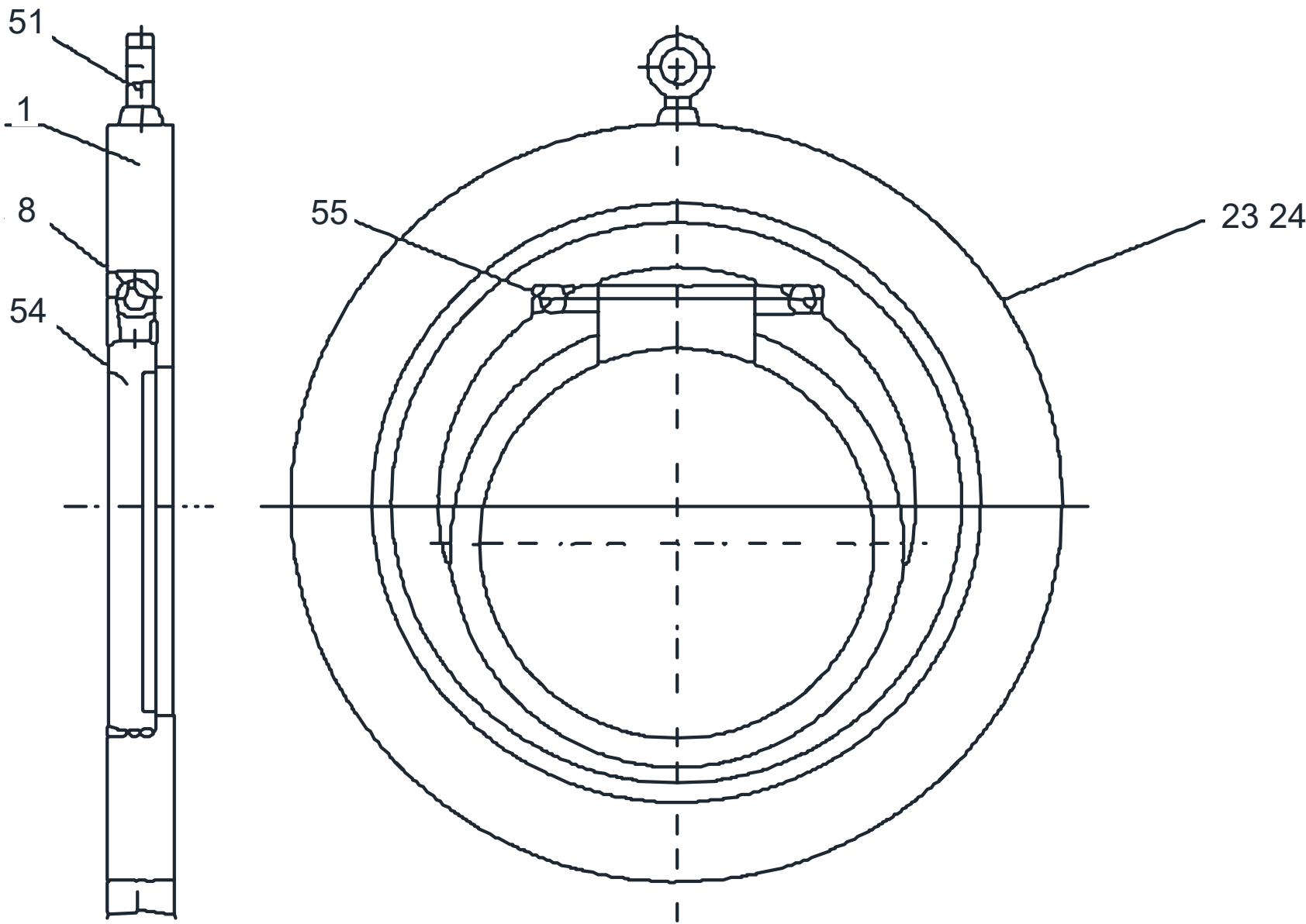
断面図
