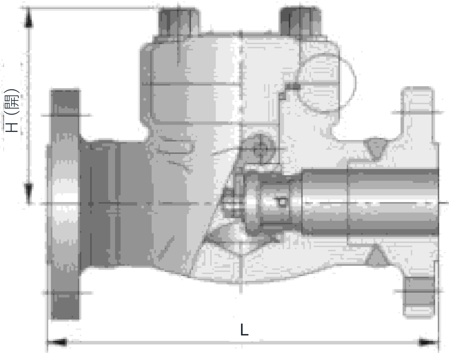
断面図
