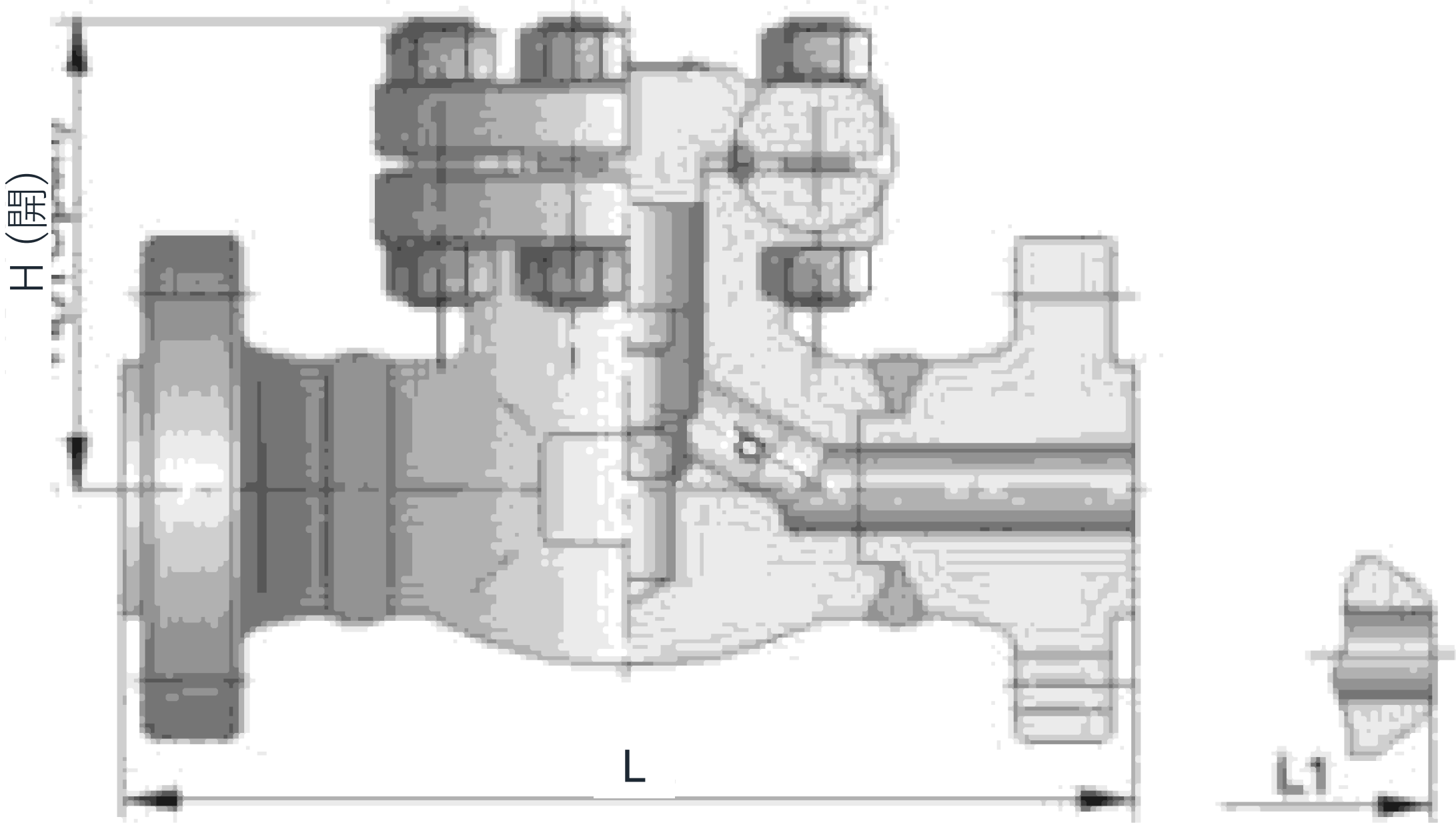
断面図
