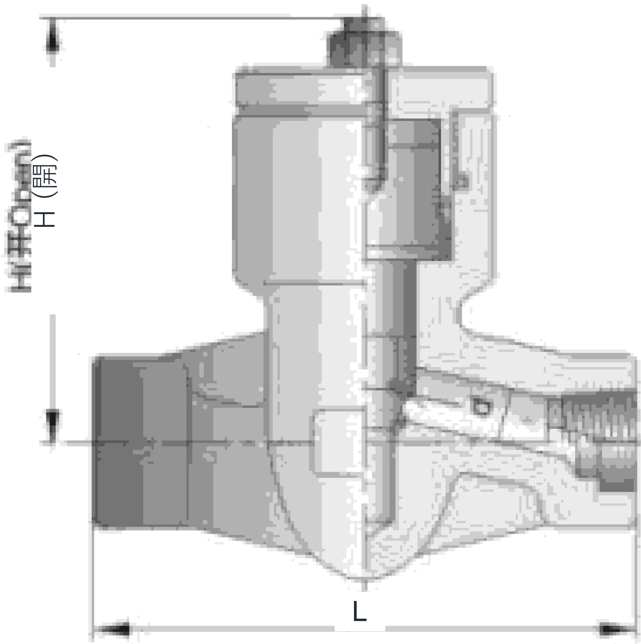
断面図
