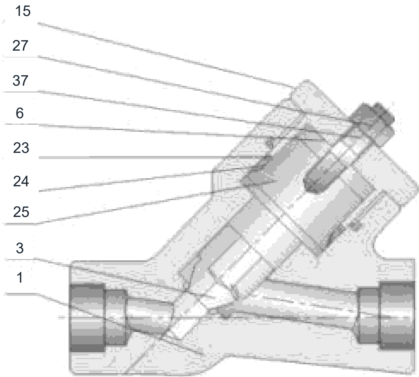
断面図
