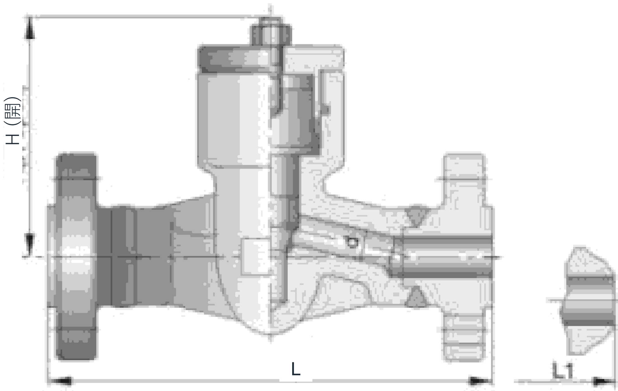
断面図
