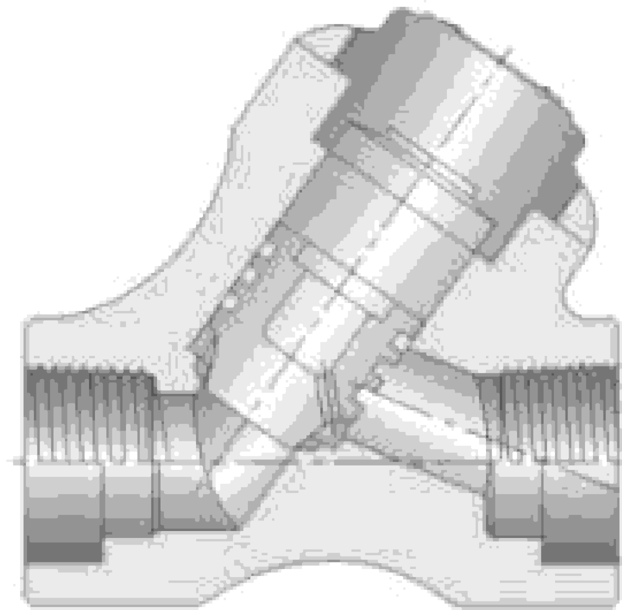
断面図
