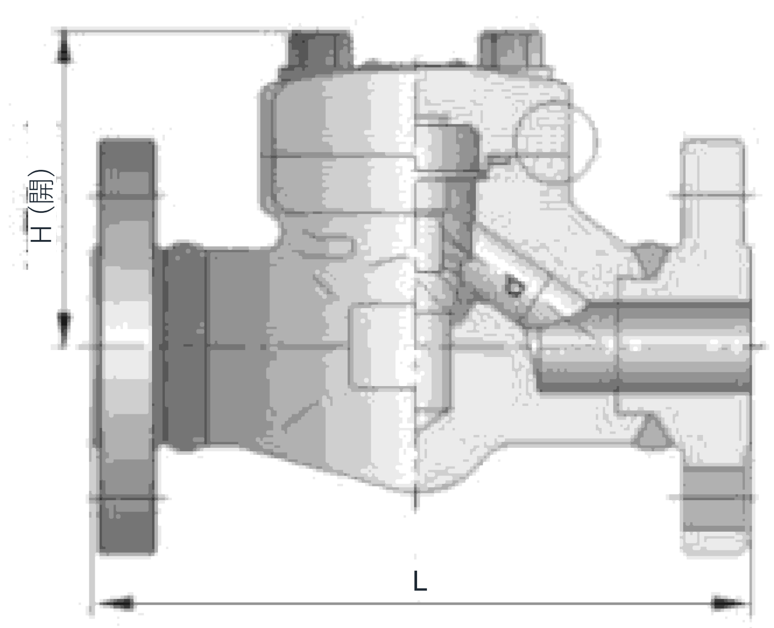
断面図
