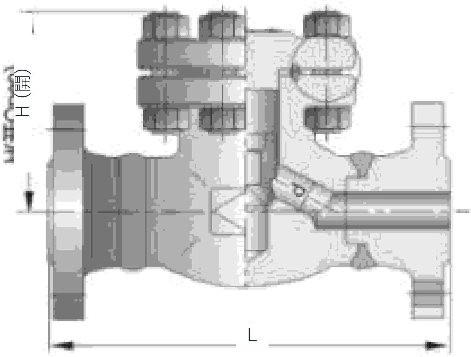
断面図
