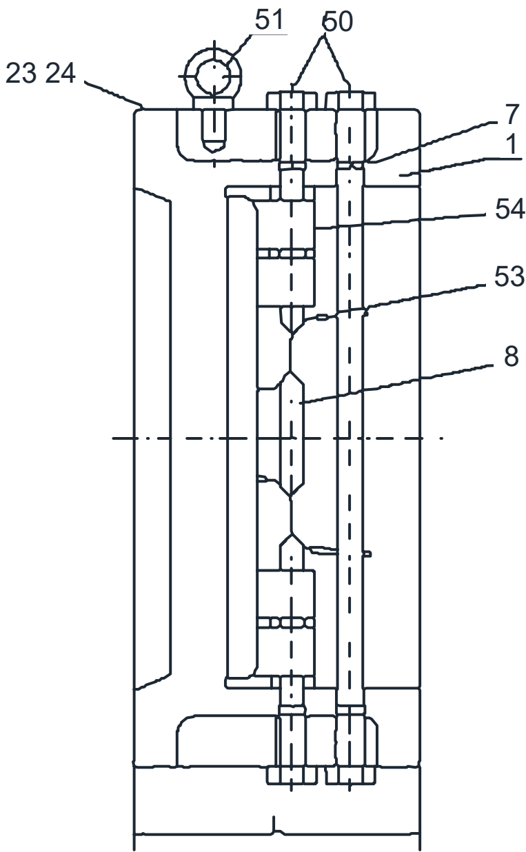
断面図
