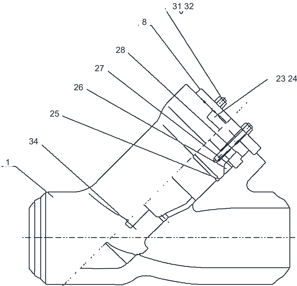
断面図
