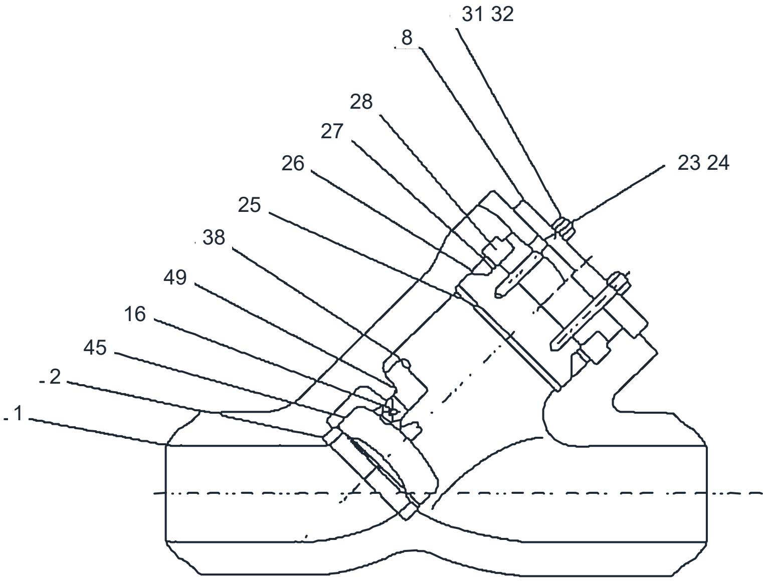
断面図
