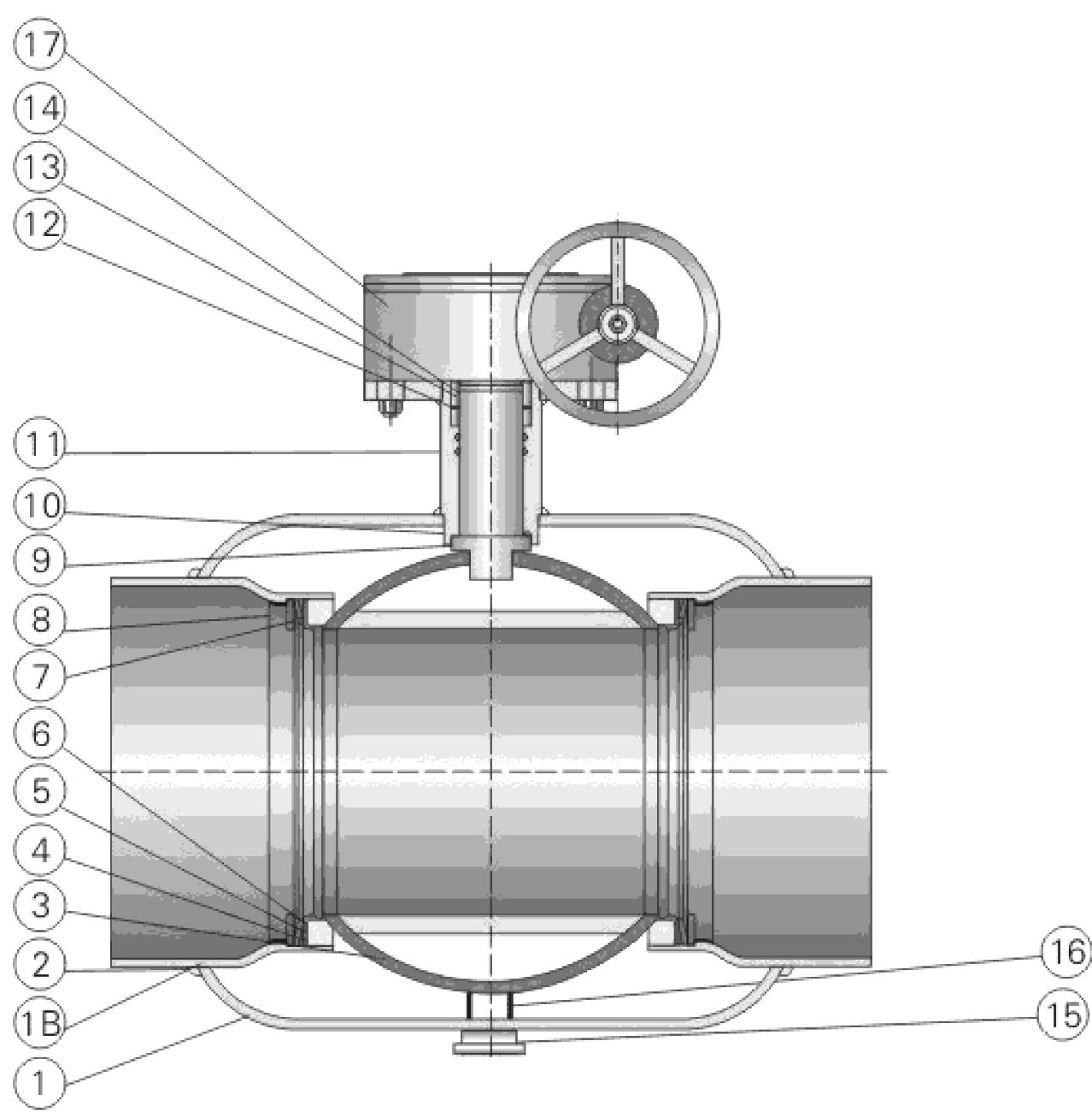
断面図
